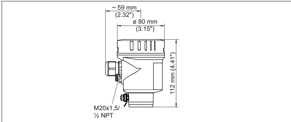
Fig. 23: Variantes de carcasa en grado de protección IP 66/IP 68; (0,2 bar), (con módulo de visualización y configuración integrado aumenta la altura de la carcasa en 9 mm/0.35 in)
