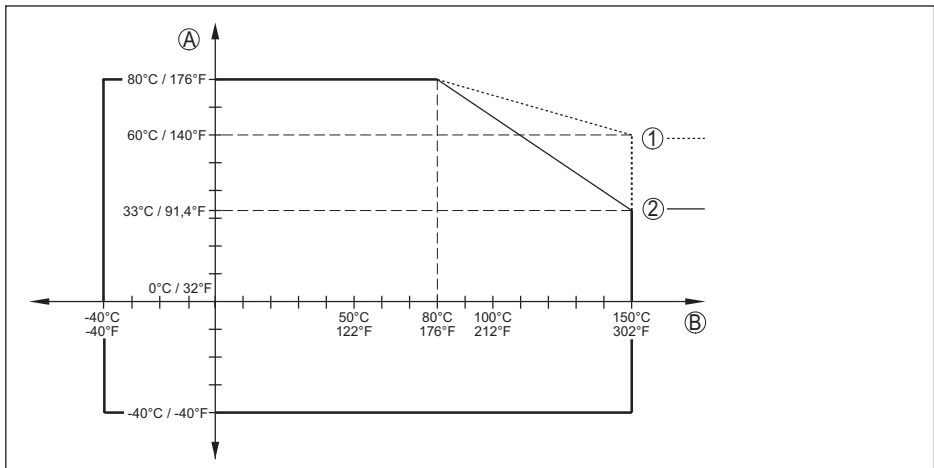
Fig. 20: Temperatura ambiente - Temperatura de proceso, versión estándar
