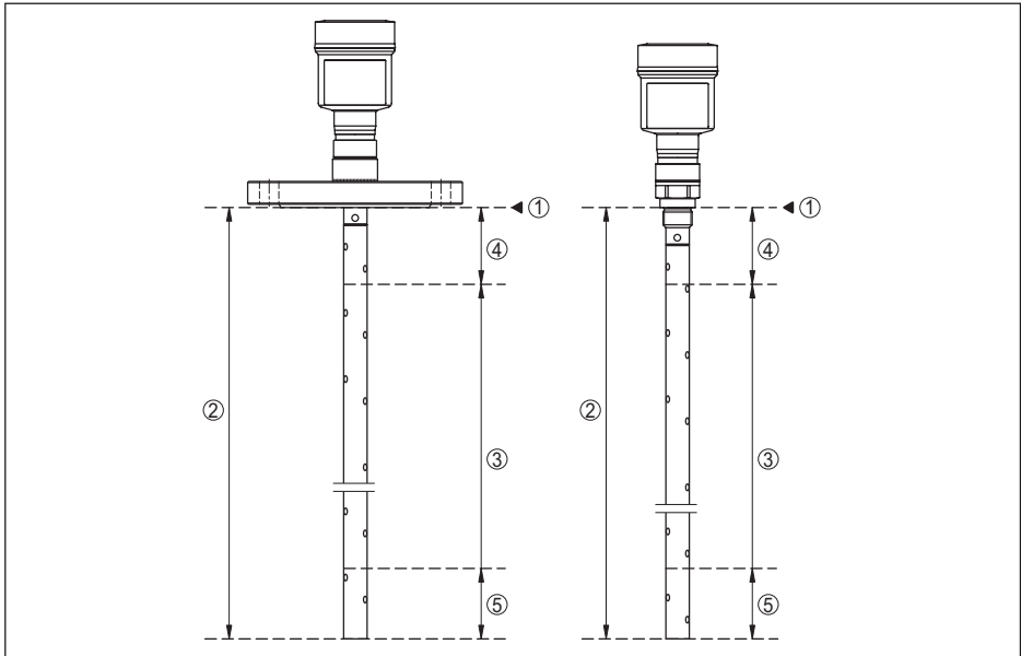
Fig. 17: Rangos de medida - NivoGuide 8100
