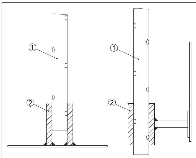
Fig. 6: Fijar la sonda de medición
