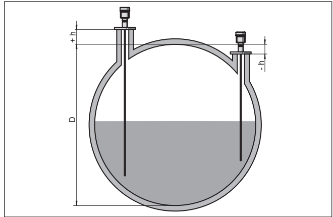
Fig. 14: Altura del depósito y valor de corrección de tubuladura
