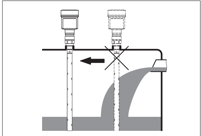
Fig. 5: Montaje del sensor en flujo de entrada de producto
