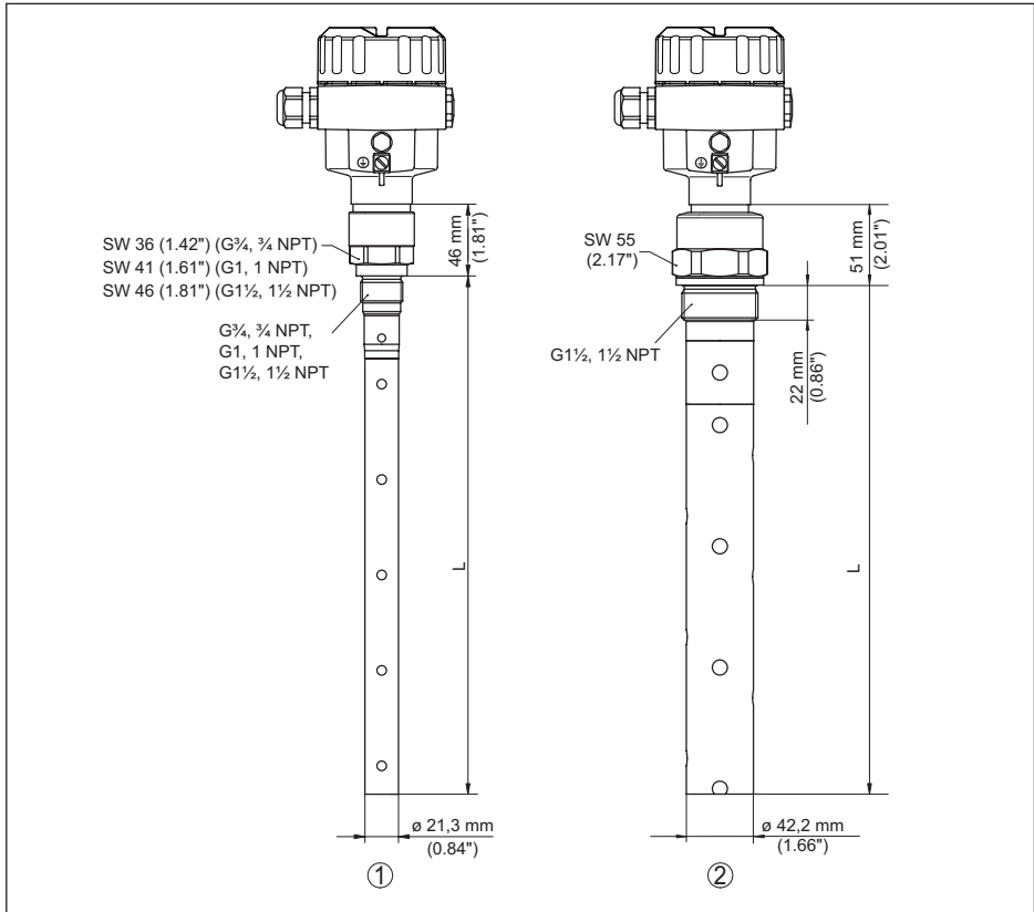
Fig. 24: NivoGuide 8100, versión roscada
