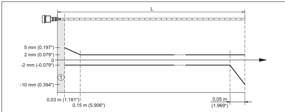
插图. 18: 同轴型 NivoGuide 8100 在介质“水”中的测量偏差
