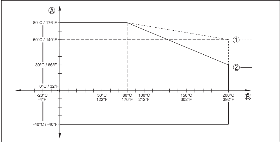
插图 21: 环境温度 - 过程温度、带有温度连接元件的类型
