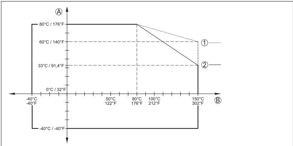
插图. 20: 环境温度 - 过程温度, 标准型
