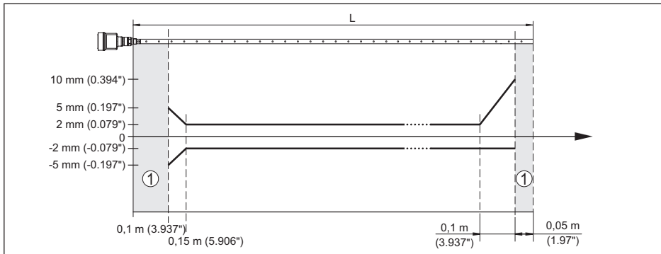
插图. 19: 同轴型 NivoGuide 8100 在介质“油”中的测量偏差
