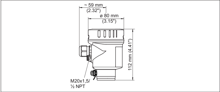
插图. 23: 采用保护等级达 IP 66/IP 68 (0.2 bar) 的壳体型式, (内装显示和调整模块后, 壳体高度增加了 9 mm/0.35 in)
