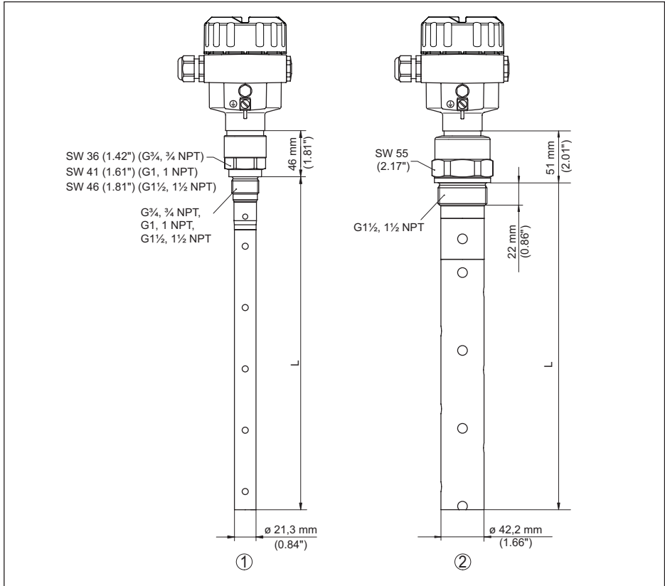
插图. 24: NivoGuide 8100, 螺纹型
