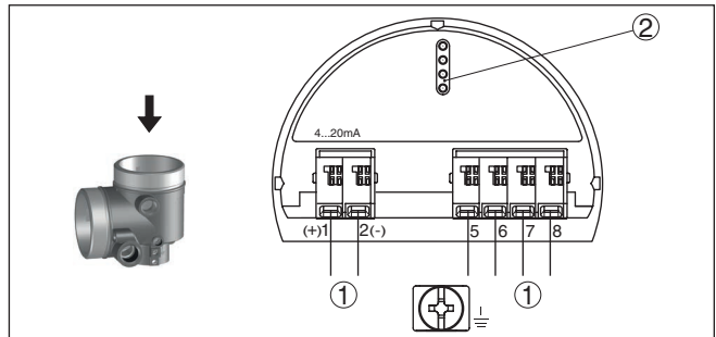
插图 9: 双腔式壳体的电子部件腔
