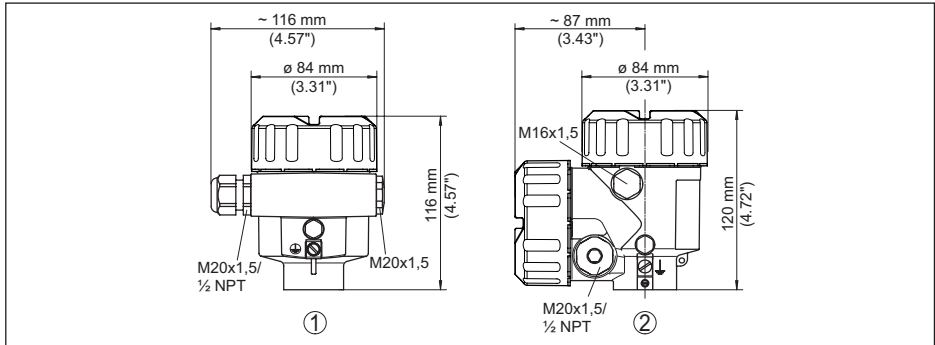
插图. 22: 采用保护等级达 IP 66/IP 68 (0.2 bar) 的壳体型式, (内装显示和调整模块后, 壳体高度增加了 9 mm/0.35 in)
