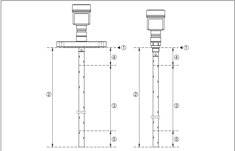
插图 17: NivoGuide 8100 的测量范围
