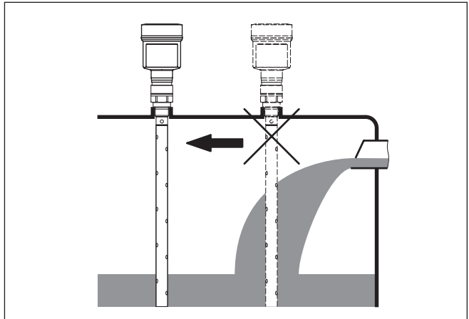
插图. 5: 流入介质时安装传感器
