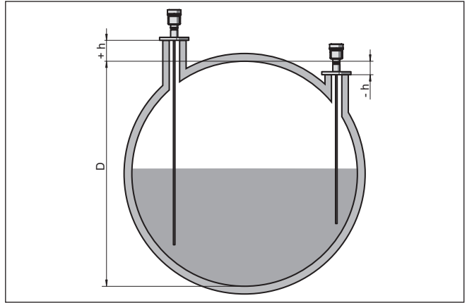
插图. 14: 容器高度和套管修正值
