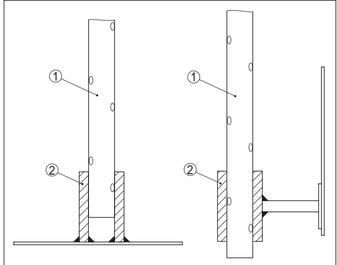
插图. 6: 将测量探头固定好
