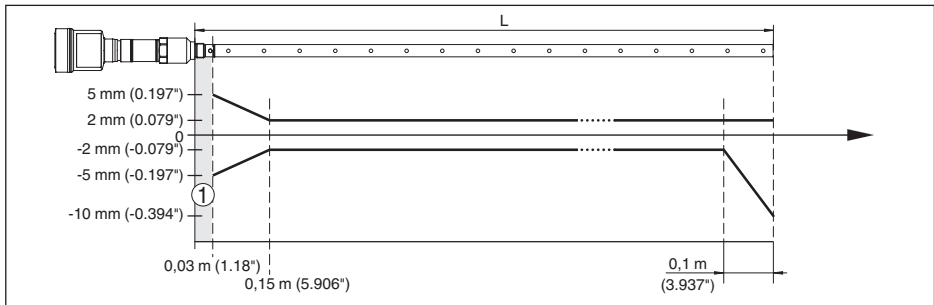
Fig. 19: Error de medición NivoGuide 8200 en versión coaxial en producto agua (longitud de medición hasta 1,5 m/4.92 ft)
