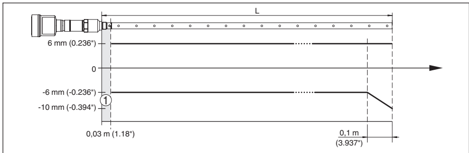
Fig. 20: Error de medición NivoGuide 8200 en versión coaxial en producto agua (longitud de medición hasta 6 m/19.69 ft)
