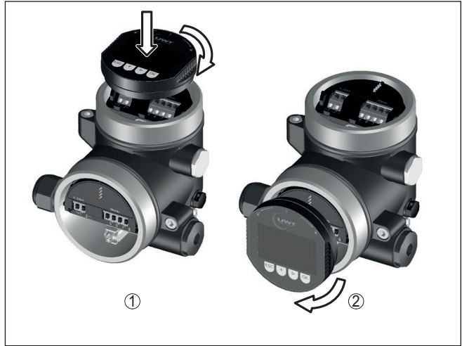
Fig. 13: Empleo del módulo de visualización y configuración en carcasa de dos cámaras
