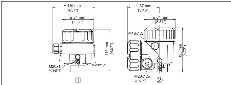
Fig. 24: Variantes de carcasa en grado de protección IP 66/IP 68; (0,2 bar), (con módulo de visualización y configuración integrado aumenta la altura de la carcasa en 9 mm/0.35 in)
