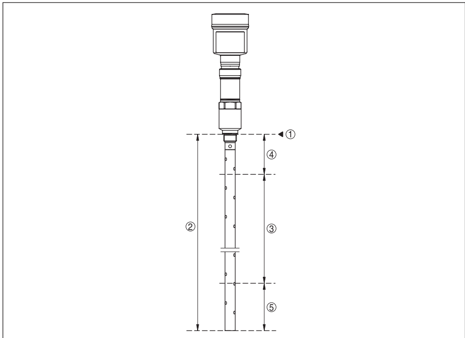
Fig. 18: Rangos de medida - NivoGuide 8200
