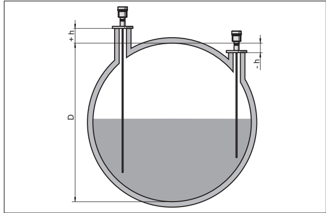
Fig. 15: Altura del depósito y valor de corrección de tubaladura
