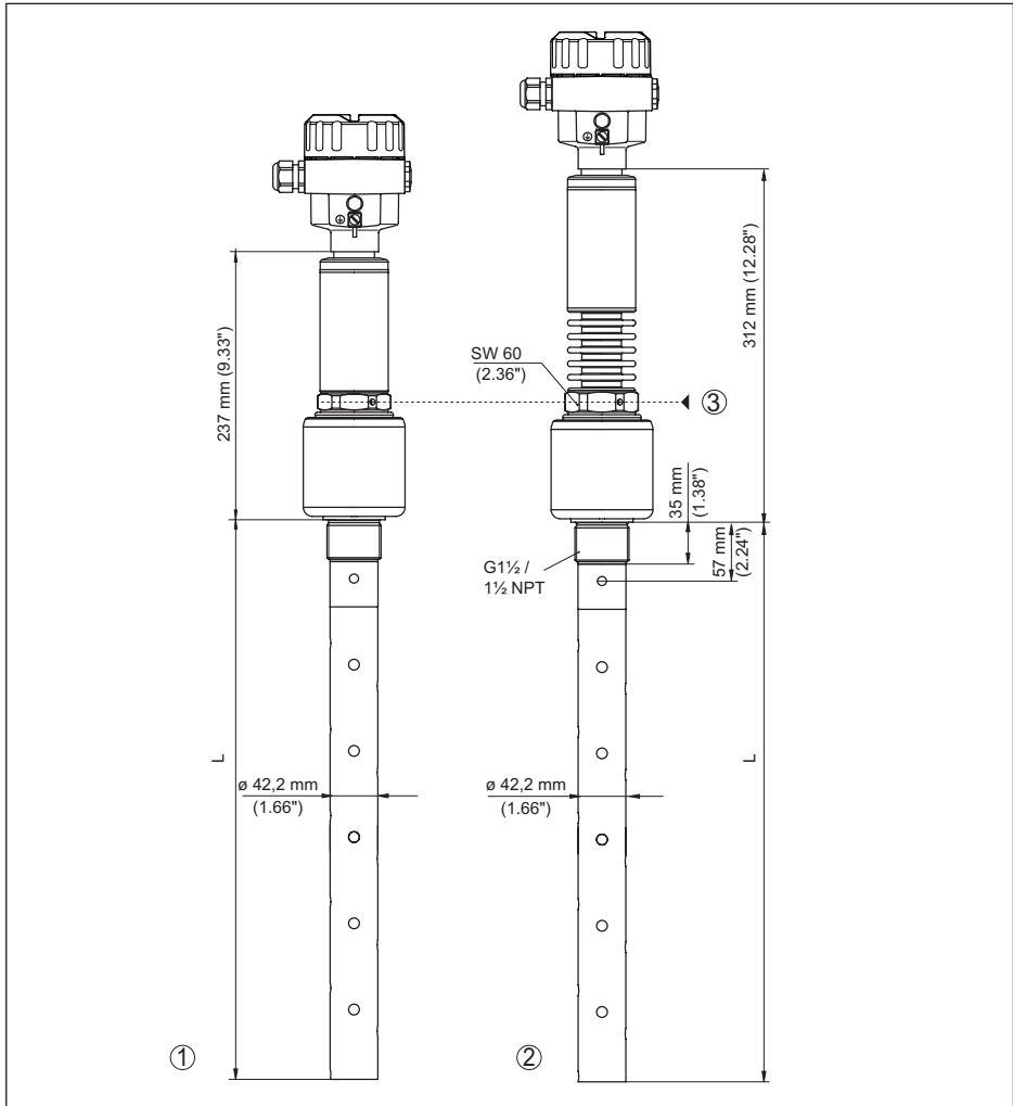
Fig. 37: NivoGuide 8200, Modelo com rosca
