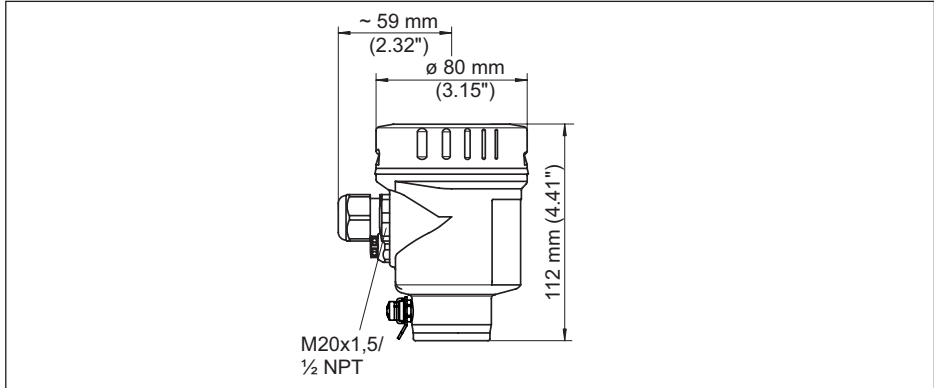
Fig. 35: Variantes da caixa com grau de proteção IP 66/IP 68, (0,2 bar), (com o módulo de visualização e configuração montado, a altura da caixa é aumentada em 9 mm/0,35 in)
