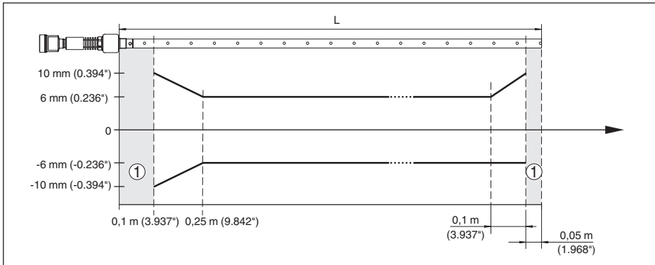
Fig. 28: Diferença de medição NivoGuide 8200 em modelo coaxial no produto óleo (comprimento de medição até 6 m/19.69 ft)
