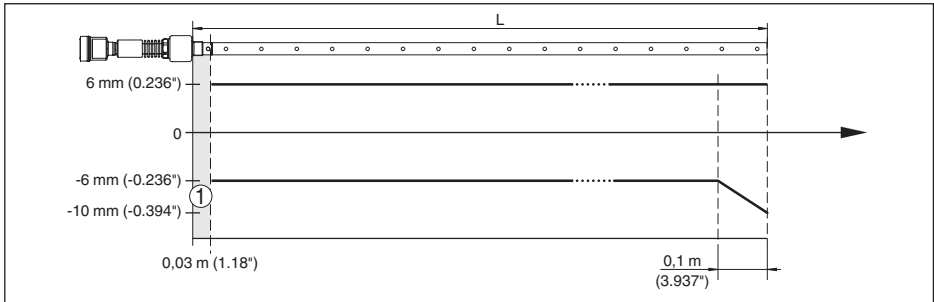
Fig. 21: Diferença de medição NivoGuide 8200 em modelo coaxial no produto água (Comprimento de medição até 6 m/19.69 ft)
