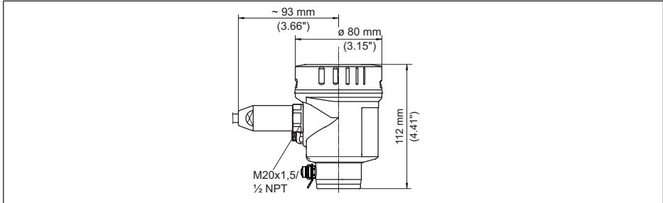
Abb. 27: Gehäuseausführungen in Schutzart IP 66/IP 68 (1 bar), (mit eingebautem Anzeige- und Bedienmodul vergrößert sich die Gehäusehöhe um 9 mm/0.35 in)
