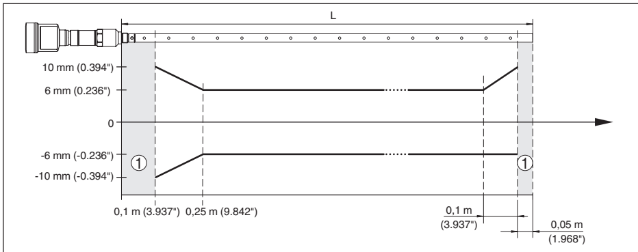
Abb. 22: Messabweichung NivoGuide 8200 in Koaxialausführung in Medium Öl (Messlänge bis 6 m/19.69 ft)
