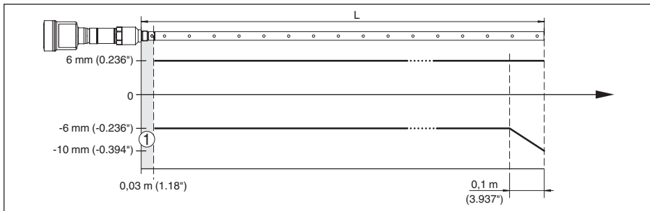
Abb. 20: Messabweichung NivoGuide 8200 in Koaxialausführung in Medium Wasser (Messlänge bis 6 m/19.69 ft)
