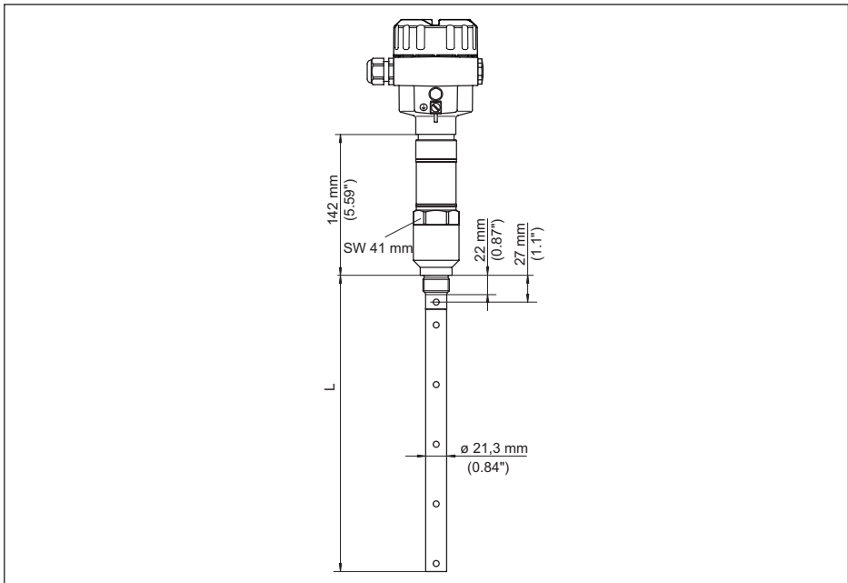
Abb. 28: NivoGuide 8200, Koaxialausführung mit Gewinde (-20 ... +250 °C/-4 ... +482 °F)
