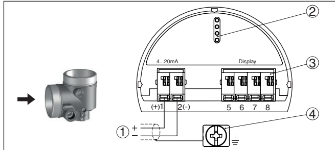
Abb. 11: Anschlussraum - Zweikammergehäuse
