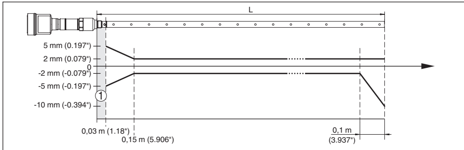
Abb. 19: Messabweichung NivoGuide 8200 in Koaxialausführung in Medium Wasser (Messlänge bis 1,5 m/4.92 ft)
