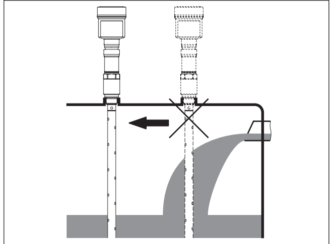
Abb. 5: Montage des Sensors bei einströmendem Medium
