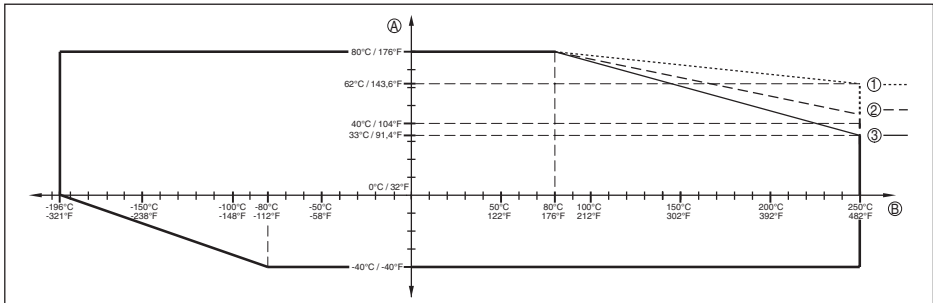
Abb. 23: Umgebungstemperatur - Prozesstemperatur, Standardausführung
