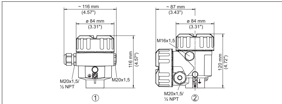
Abb. 24: Gehäuseausführungen in Schutzart IP 66/IP 68 (0,2 bar), (mit eingebautem Anzeige- und Bedienmodul vergrößert sich die Gehäusehöhe um 9 mm/0.35 in)
