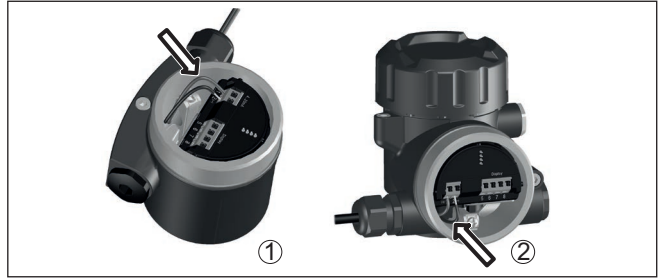
插图. 3: 接线步骤5和6
