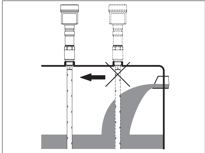
Fig. 5: Montagem do sensor no fluxo de entrada do produto
