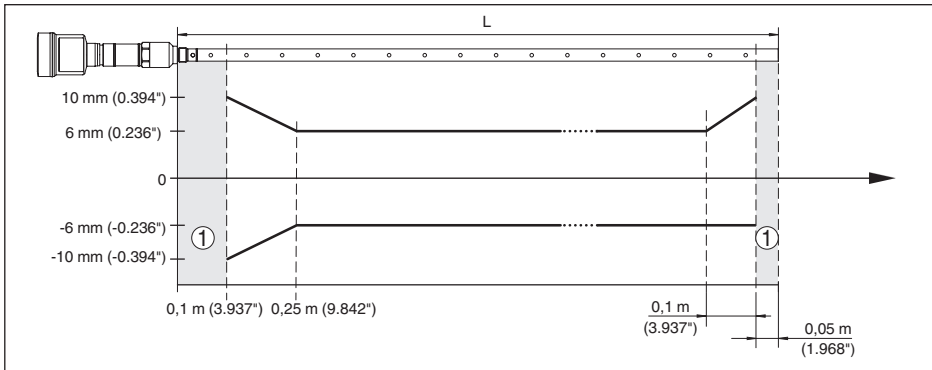
Fig. 22: Diferença de medição NivoGuide 8200 em modelo coaxial no produto óleo (comprimento de medição até 6 m/19.69 ft)
