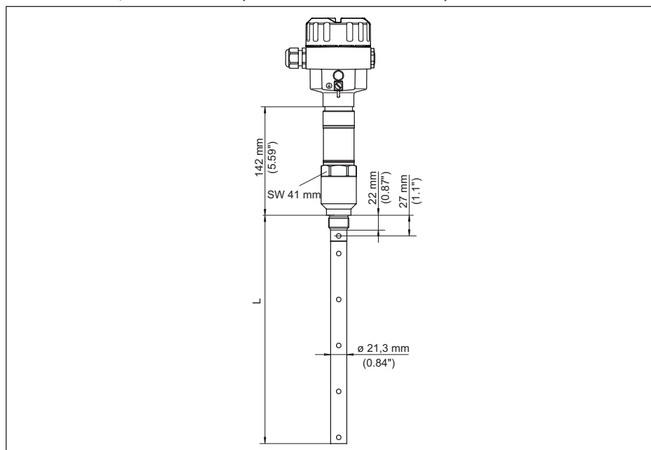
Fig. 28: NivoGuide 8200, modelo coaxial com rosca (-20 ... +250 °C/-4 ... +482 °F)
