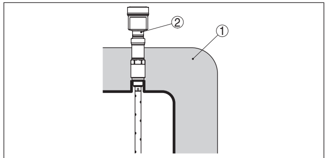
Fig. 7: Montagem do aparelho em reservatórios isolados.
