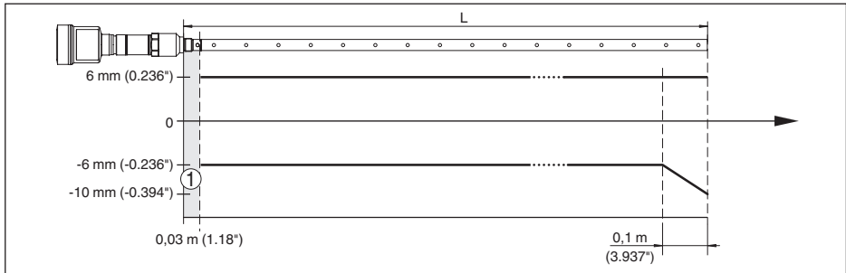
Fig. 20: Diferença de medição NivoGuide 8200 em modelo coaxial no produto água (Comprimento de medição até 6 m/19.69 ft)
