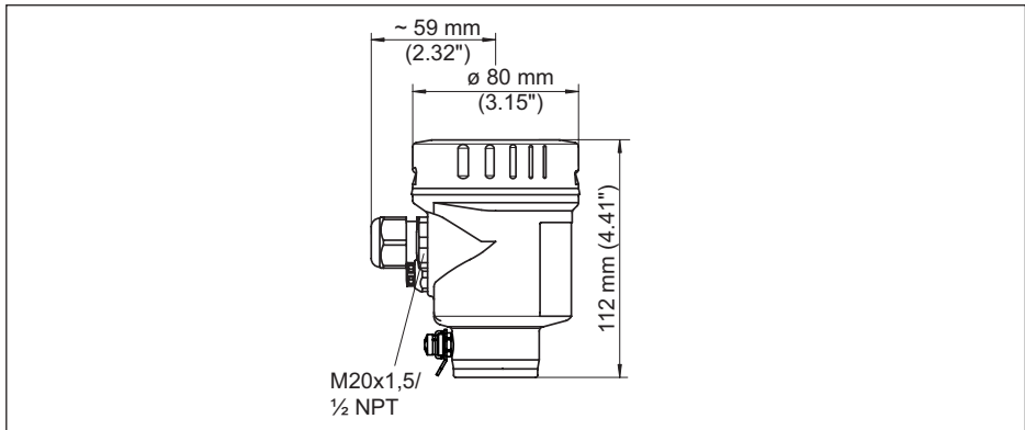
Fig. 26: Variantes da caixa com grau de proteção IP 66/IP 68, (0,2 bar), (com o módulo de visualização e configuração montado, a altura da caixa é aumentada em 9 mm/0,35 in)
