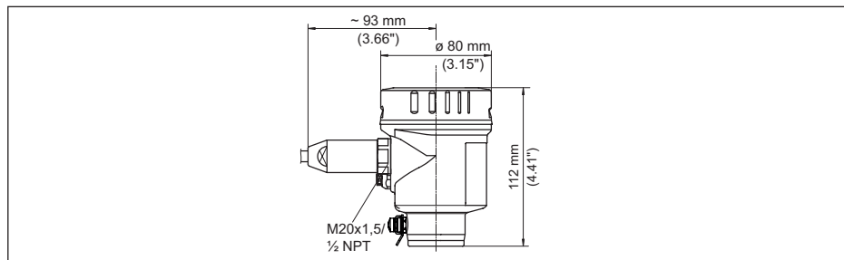
Fig. 27: Variantes da caixa com classe de proteção contra corpos estranhos e umidade com grau de proteção IP 66/IP 68, (1 bar), (com o módulo de visualização e configuração montado, a altura da caixa é aumentada em 9 mm/0,35 in)
