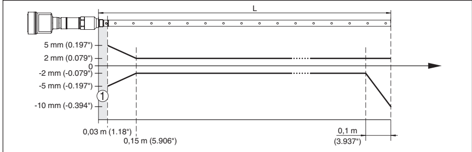
Fig. 19: Diferença de medição NivoGuide 8200 em modelo coaxial no produto água (Comprimento de medição até 1,5 m/4.92 ft)
