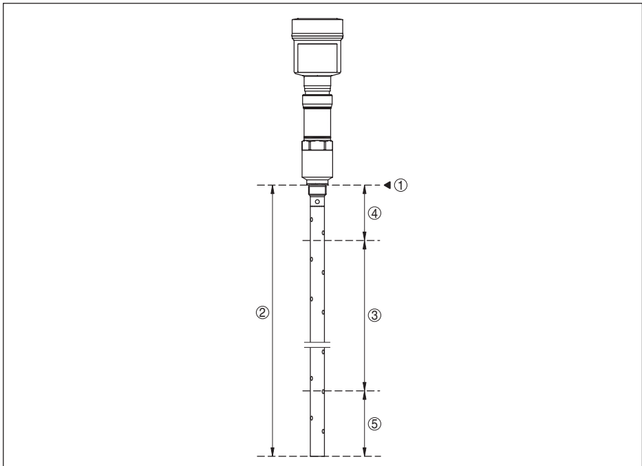
Fig. 18: Faixas de medição - NivoGuide 8200
