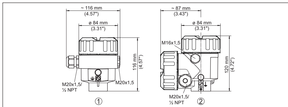
Fig. 24: Variantes da caixa com grau de proteção IP 66/IP 68, (0,2 bar), (com o módulo de visualização e configuração montado, a altura da caixa é aumentada em 9 mm/0,35 in)
