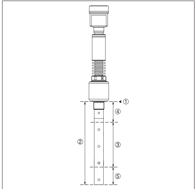
Fig. 8: Plages de mesure - NivoGuide 8200
